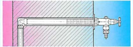
Abbildung II: Bestell-Nr. 7000 - 7025 Frostsichere Auslaufarmatur mit Steckschlüssel, kurze Ausführung, für Wanddicken von 150 mm bis 300 mm, Zuleitung unter Putz.
