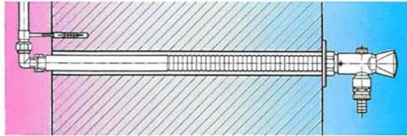
Abbildung I: Bestell-Nr. 7050 - 7075 Frostsichere Auslaufarmatur mit Dreikantgriff, lange Ausführung, für Wanddicken von 250 mm bis 500 mm, Wasser-Zuleitung innen auf Putz.
