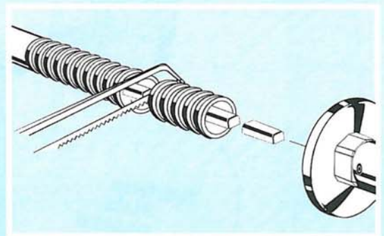
Abbildung II: Bestell-Nr. 7000 - 7025 Frostsichere Auslaufarmatur mit Steckschlüssel, kurze Ausführung, für Wanddicken von 150 mm bis 300 mm, Zuleitung unter Putz.
