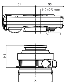
Variante déportée Type IST, TE1, M60, PCC
