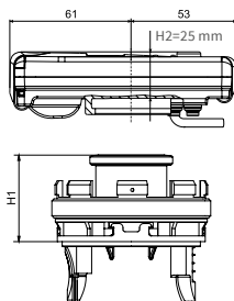
Variante déportée Type ASF A1
