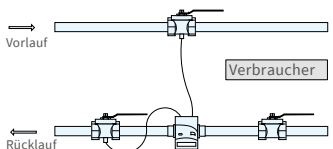
Symmetrischer Fühlereinbau bei zelsius® C5-CMF
