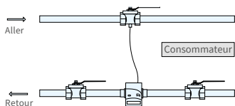
Installation de la sonde asymétrique pour zelsius® C5-CMF avec sonde retour intégrée dans le mesureur
