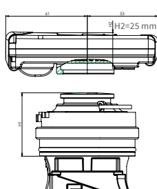
Variante Combi tipo A1
