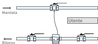
Installazione asimmetrica della sonda per zelsius® con sonda di ritorno integrata nel corpo.
