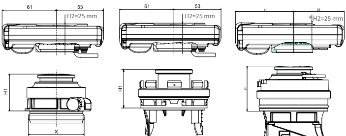
Kombivariante Typ IST, TE1, M60, PCC
