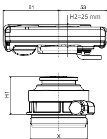
Variante Combi tipo IST, TE1, M60, PCC
