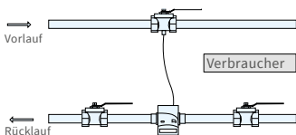
Asymmetrischer Fühlereinbau bei zelsius® C5-CMF mit Temperaturfühler im DFS integriert
