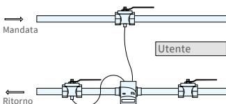
Installazione simmetrica della sonda di temperatura nel zelsius®.
