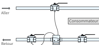
Installation de la sonde symétrique pour zelsius® C5-CMF
