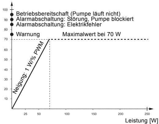
Abb. 8 PWM-Rückmeldesignal - Leistungsaufnahme
