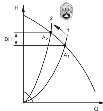
Abb. 16 Unregelte Pumpe
