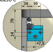
DETTAGLIO C
