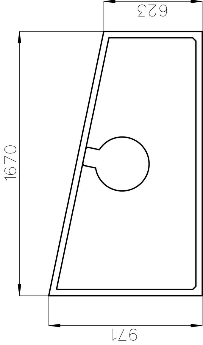
Draufsicht
