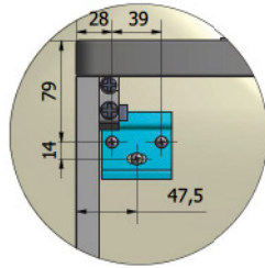
DETTAGLIO B
