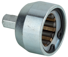
1x S-Anschluss-Montagewerkzeug Zum Ein- und Ausdrehen von S-Anschlüssen für Aufputz-Wandarmaturen
