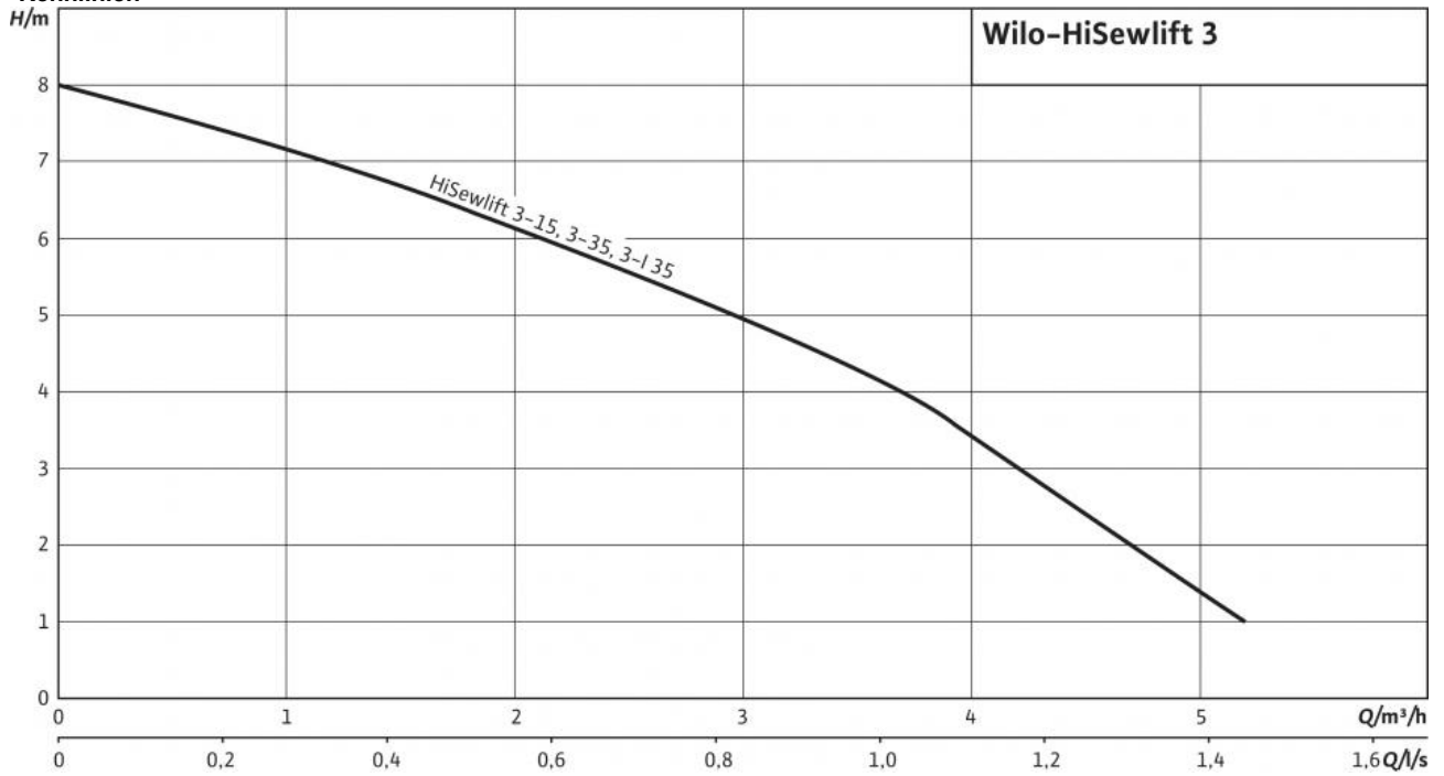
Kennlinien
