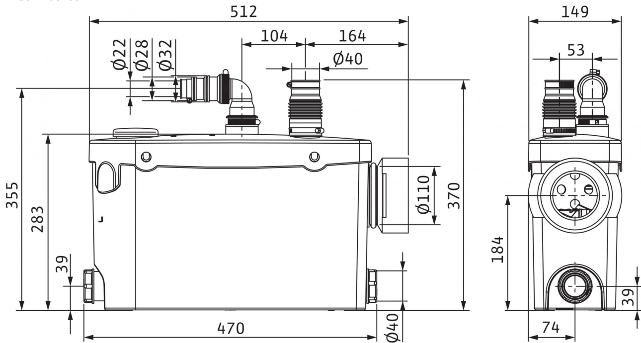
Maßzeichnung HiSewlift 3-I35 HiSewlift 3-I35
